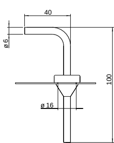
Climaset® 6550/6556
